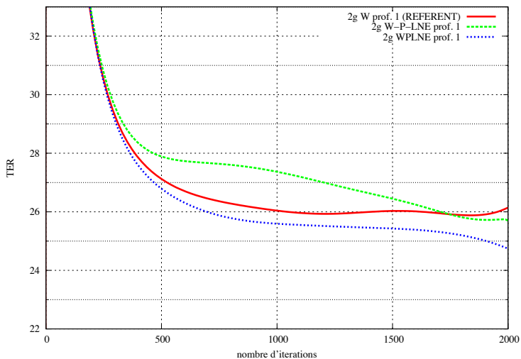
FIGURE 1 – Comparaison des performances des différents niveaux Ngrammes TEXT pour le système TEXT(2g)+SNA+SPONTA
