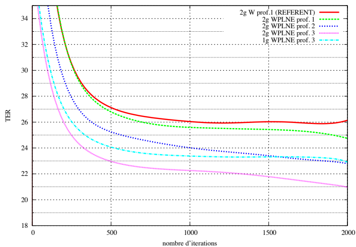
FIGURE 2 – Courbes de résultats pour différentes configurations de profondeur de bonzaïs et de descripteurs en fonction du nombre d'itération de boosting).
