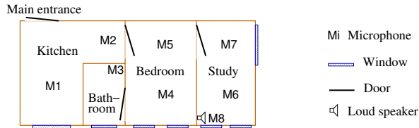
FIGURE 2 – Position des microphones dans l'appartement domus
