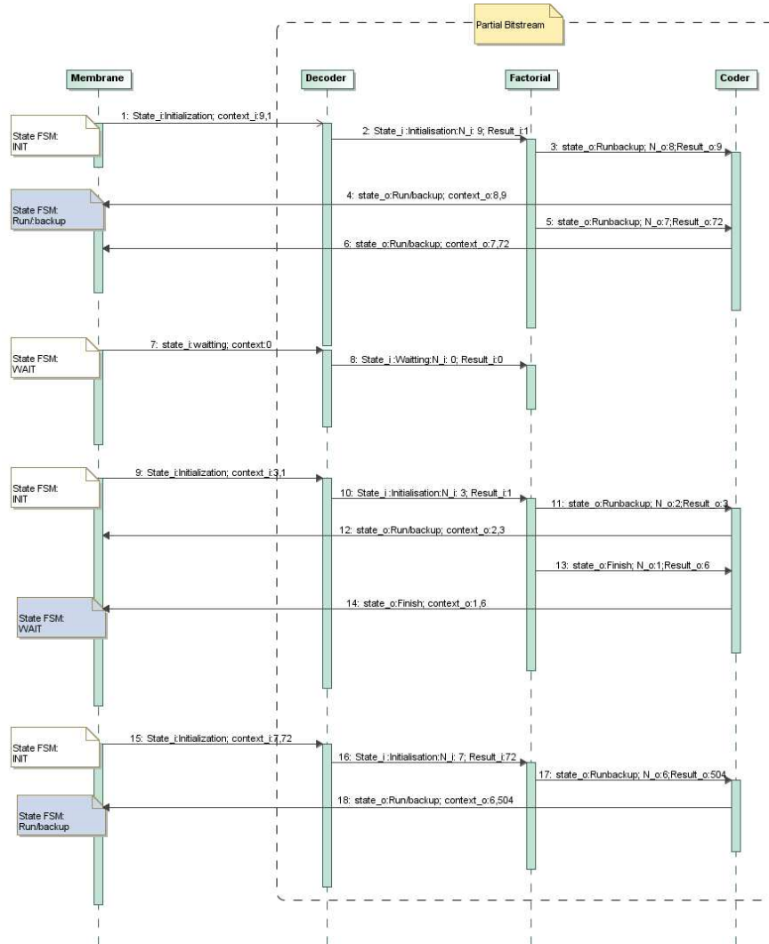
FIGURE 7 – Diagramme UML d’une simulation de calculs factoriels
