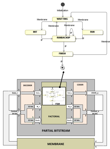
FIGURE 6 – Architecture à base de membrane pour une application factorielle reconfigurable
