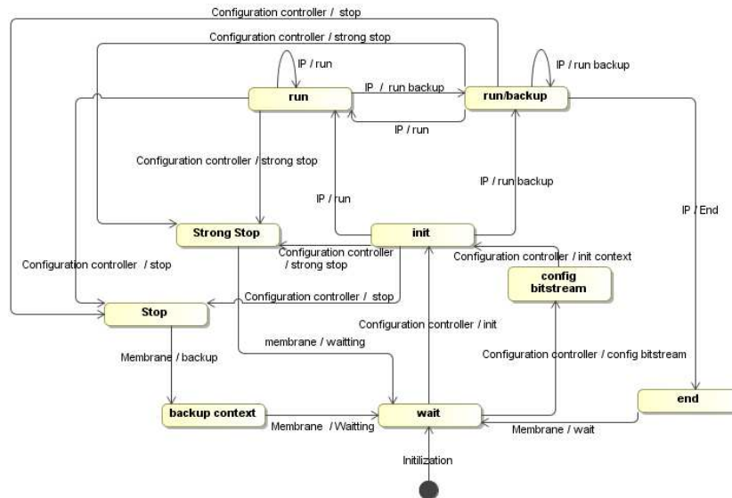
FIGURE 5 – Diagramme UML de la FSM du composant virtuel
