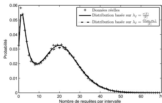
FIGURE 2: Distribution du nombre de débuts de sessions par intervalle de cinq minutes (traces et modèles).
