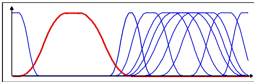
Figure 19 : Solutions de la forme \zeta m_\beta P \grave{E} avec \rho^* = 0.3
