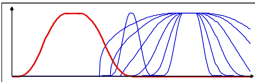
Figure 20 : Solutions de la forme \zeta f_x P \grave{E} avec \rho^* = 0.3
