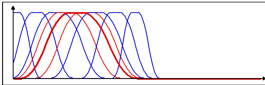
Figure 13 : Propriétés \zeta assez similaires \square A de la forme \zeta m_\alpha A \hat{E}
