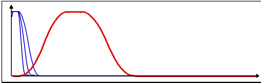
Figure 18 : Solutions de la forme \zeta f_x m_\beta A \grave{E} avec \rho^* = 0.3
