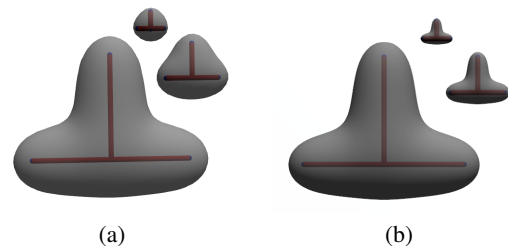
Figure 7: Application d'une homothétie à la fois aux dimensions d'un squelette de convolution et aux poids \tau associés. La formulation classique (a) ne génère pas des formes similaires contrairement à la formulation homothétique (b). Le noyau utilisé est Cauchy 4 avec \sigma = \frac{1}{2} . Pour (a), on a \tau = 14 pour la forme la plus grande, pour (b), on a \tau = 1 . Le rapport de la première homothétie est \frac{1}{3} , celui de la seconde est \frac{1}{2} .
