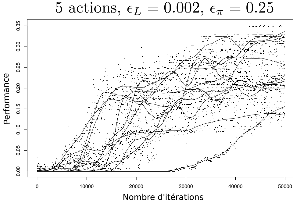
FIGURE 7 – Apprentissage avec 5 actions, les points représentent les performances mesurées toutes les 100 itérations sur 10 trajectoires, chaque trajectoire est représentée en étant lissée.
