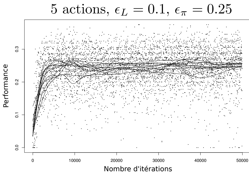
FIGURE 5 – Apprentissage avec 5 actions, les points représentent les performances mesurées toutes les 100 itérations sur 10 trajectoires, chaque trajectoire est représentée en étant lissée.
