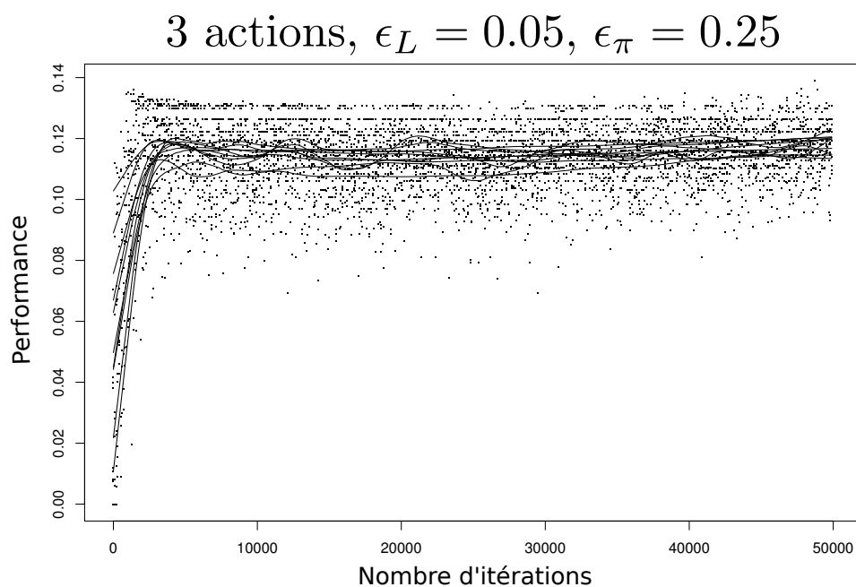
FIGURE 4 – Apprentissage avec 3 actions, les points représentent les performances mesurées toutes les 100 itérations sur 10 trajectoires, chaque trajectoire est représentée en étant lissée.
