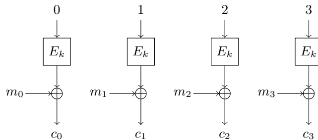
Fig. 1. CTR mode
