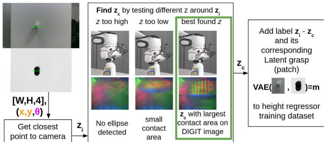
FIGURE 4.8 – Trouver la meilleure hauteur de saisie : 5 hauteurs sont essayées pour chaque saisie 3D, la hauteur associée au plus haut \epsilon pour les deux DIGITs est retenue. La meilleure hauteur et sa saisie, encodée par le VAE de [56], est sauvegardée dans un jeu de données utilisé pour entraîner le régresseur de hauteur.
