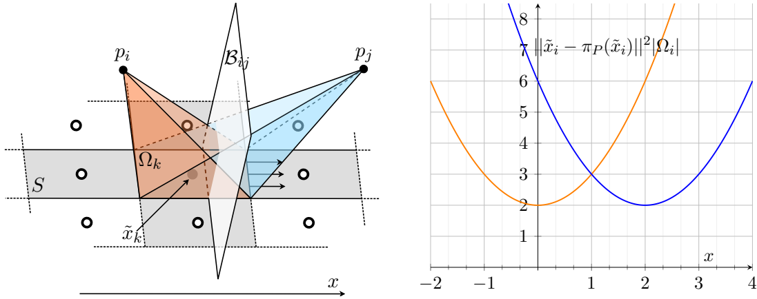
FIGURE 4.5 – À gauche : un échantillon \tilde{x}_k et sa cellule associée \Omega_k , le plus proche voisin de la cellule, p_i ou p_j varie en fonction du déplacement de la surface S sur l'axe x . Les points p_i et p_j définissent un plan médiateur \mathcal{M}_{ij} si \tilde{x}_k \in \mathcal{M}_{ij} le plus proche voisin de \tilde{x}_k n'est pas unique. À droite : mesure de l'erreur de l'échantillon \tilde{x}_k au point p_i en orange et à p_j en bleu, le minimum de ces deux fonctions est notre fonction d'énergie. La fonction n'est pas dérivable à l'intersection des deux courbes.
