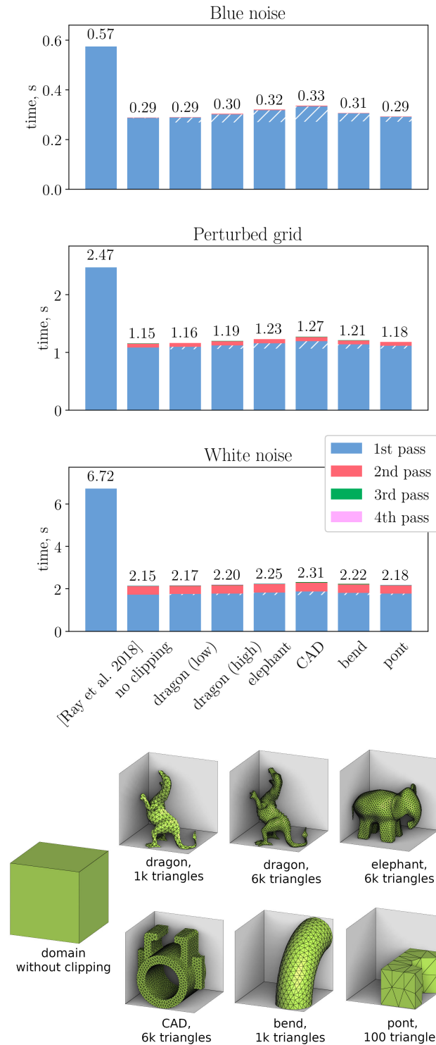
FIGURE 3.13 – Statistiques sur 10M racines de Voronoï avec distribution de bruit bleu (en haut), situées sur une grille perturbée (milieu) et bruit blanc (en bas). La colonne la plus à gauche correspond au temps d'exécution de l'algorithme [Ray et al., 2018]; la deuxième colonne est notre résultat sans restriction ; 6 colonnes de droite correspondent à différents domaines restreints.
