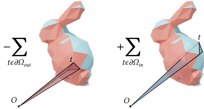
FIGURE 3.8 – Un exemple de calcul de volume : lorsque la normale du triangle t pointe vers le point O (à gauche), le volume du tétraèdre est retiré de la somme, sinon (à droite) il est ajouté.
