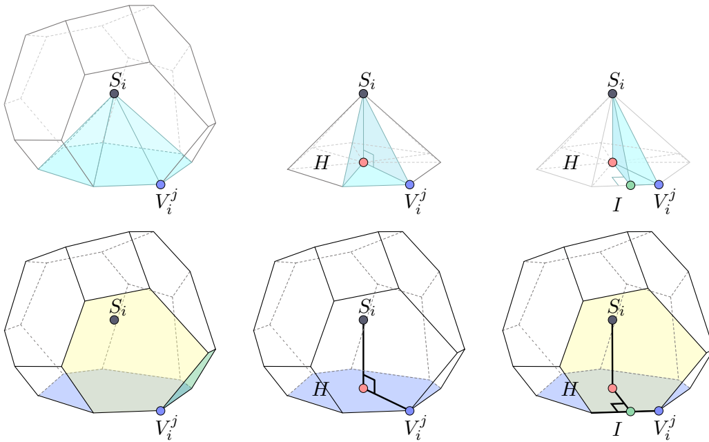
FIGURE 3.7 – Ligne supérieure : pour décomposer la cellule convexe en tétraèdres, nous la décomposons d’abord en pyramides associées à chaque face de la cellule (image de gauche). Ensuite, cette pyramide peut se décomposer en différents tétraèdres dont la base est un triangle, enfin ces tétraèdres peuvent à nouveau être subdivisés en deux. Ligne supérieure : Puisque nous utilisons une structure de données légère, il convient de retrouver ces informations à partir de la racine S_i et de l’ensemble de plans (en jaune, vert et bleu). Pour cela, nous projetons la racine S_i sur la face en bleu (point H ). Ensuite, en projetant S_i sur l’intersection des plans jaune et bleu (point I , image de droite). À partir des points V_i^j , H , S_i et I il est possible de reconstruire un tétraèdre, en reproduisant cette construction pour tous les points V_i^j , nous pouvons obtenir la décomposition présentée ci-dessus.
