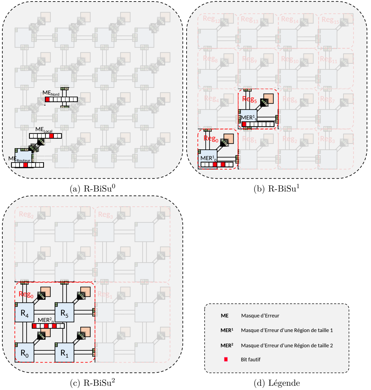
Figure 0.3: Valeurs des masques d'erreur dans un NoC défectueux avec la technique R-BiSu en considérant différentes tailles de régions.
