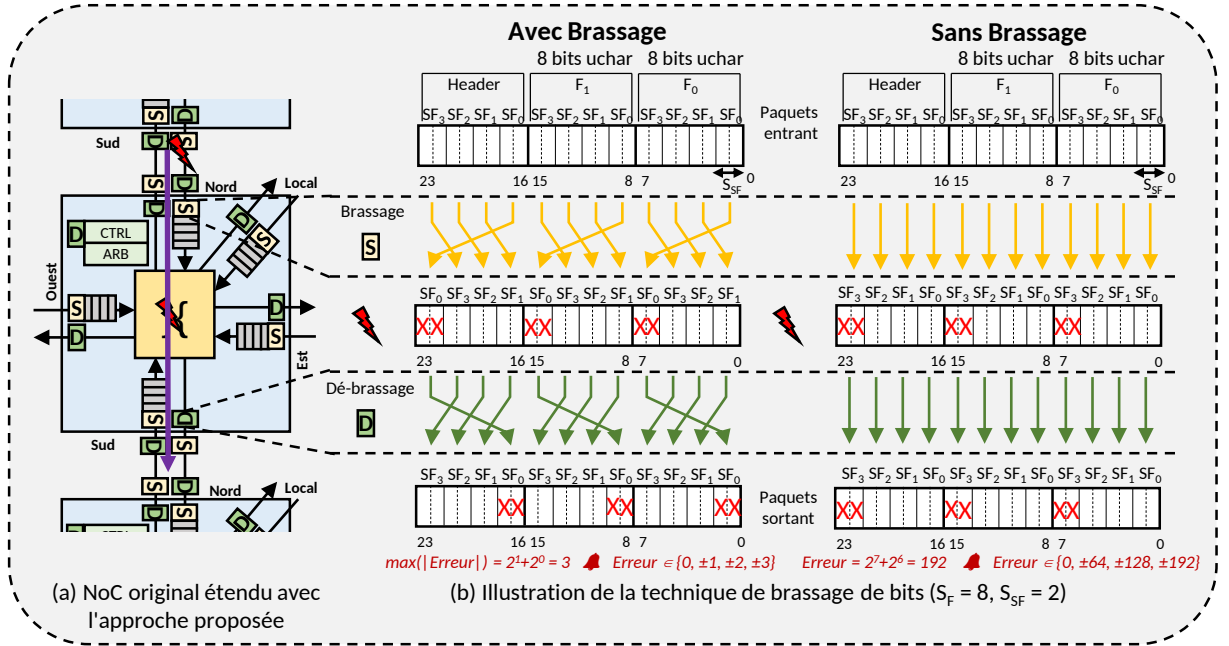
Figure 0.2: NoC classique étendu avec la technique BiSu.
