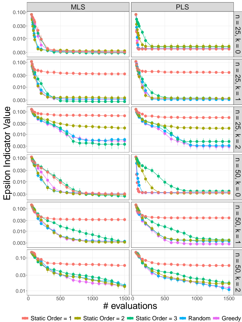
FIGURE 4.5 – Profils de convergence du framework S-MCO avec différents paramétrages de l'ordre de Walsh pour la stratégie \text{Select}_{\text{Bl}_{\text{norm}}} sur des instances de \text{mnk} -landscapes.
