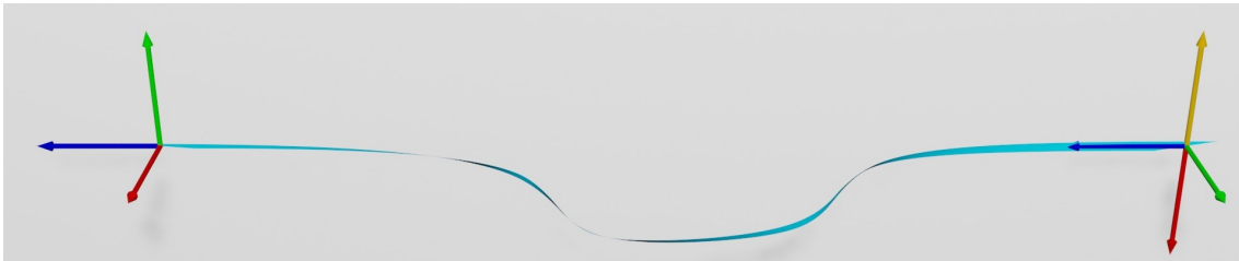
FIGURE 5.5 – Illustration de l'équilibre du ruban décrit dans le « Scénario bi-encasté » (section 5.3.2). Les encastresments sont indiqués par des flèches rouges, vertes et bleues, et la verticale par une flèche jaune. La différence entre l'utilisation de l'énergie de Sadowsky et de Wunderlich n'est pas visible à l'œil nu.
