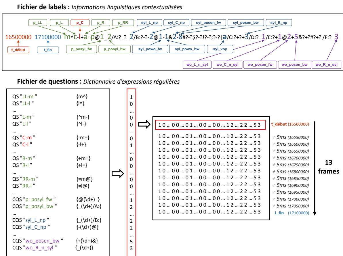
FIGURE 6.2 – Exemple illustrant la transformation de chaque ligne du fichier des labels de la figure 6.1 en séquence de vecteurs de valeurs binaires et numériques. Cette transformation se fait en respectant la durée de chaque phonème et en se basant sur la fréquence d'échantillonnage des données acoustiques.
