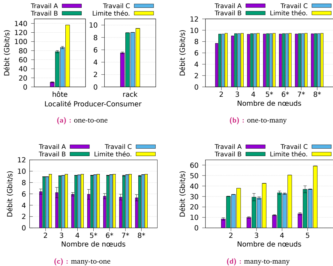
Figure 11.3 : Mesures des débits de trois travaux différents exécutés sur quatre topologies différentes par rapport aux débits maximaux (limites théoriques) de la plateforme d'évaluation
