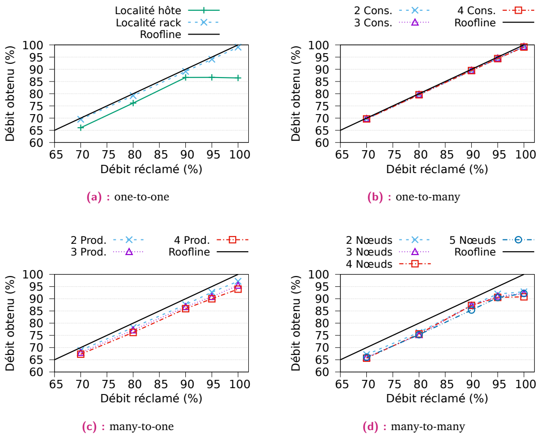
Figure 11.5 : Mesures des débits (débit obtenu) du travail B exécuté sur quatre topologies différentes en fonction d’une lecture à vitesse constante des données produites (débit réclamé). Les débits sont exprimés en pourcentage des débits obtenus pour la configuration correspondante dans la figure 11.4
