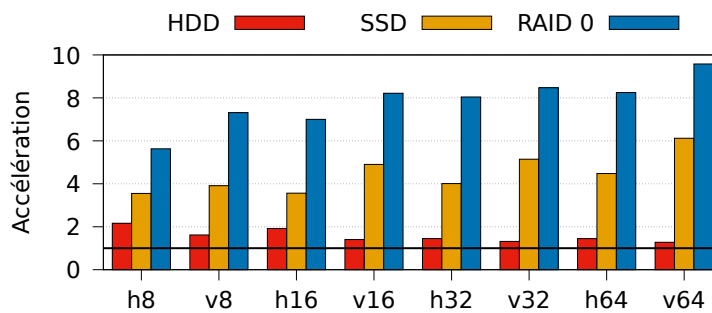
Figure 4.7 : Accélération moyenne obtenue par l’utilisation des appels systèmes posix_fadvise(3) avec une mémoire temporaire src de 1 Go sur des matrices d’orientations et de tailles différentes (de 8 Go à 64 Go)
