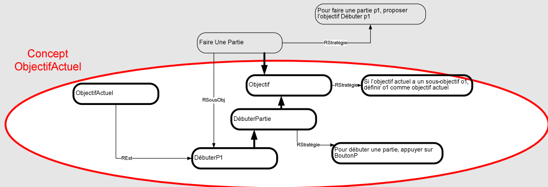
Figure 3.6 : Exemple de sous-graphe correspondant à la gestion d'un objectif
