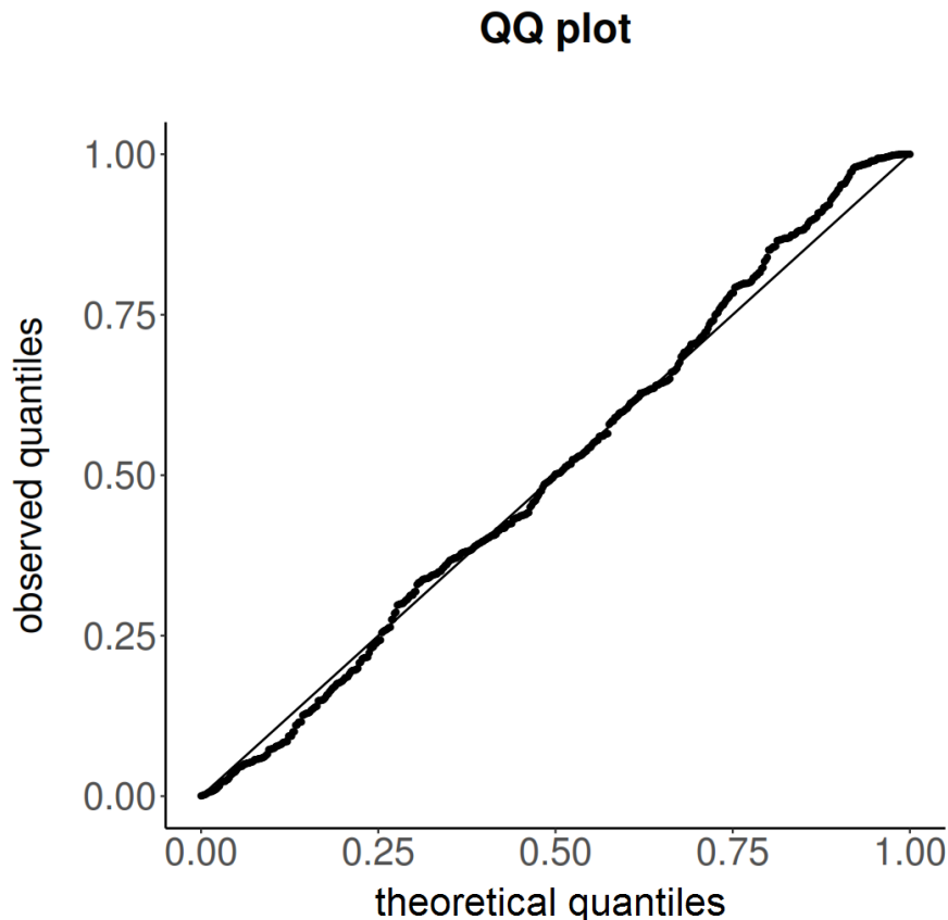
FIGURE 24 – QQ-plot des quantiles observés VS quantiles prédits avec notre méthode
