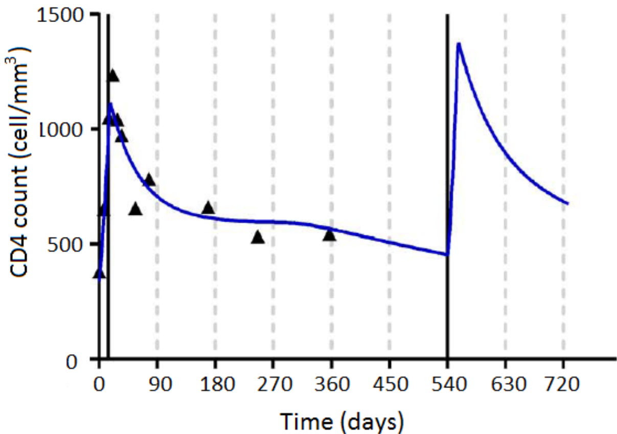
FIGURE 15 – Un des scénarios testé par [Thiébaud et al., 2014]. Les lignes grises pointillées correspondent aux temps des visites ; un nouveau cycle (ligne noire verticale) est administré lorsque le patient est sous 500 CD4 lors d'une visite. La ligne bleue correspond à la prédiction du patient selon le scénario (ici, on considère que l'effet du second cycle est le même que le premier et que l'effet sur la mort cellulaire dure entre neuf mois et deux ans)
