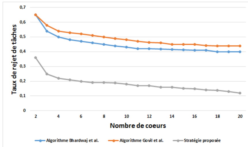
FIGURE 4.11: Taux de rejet de tâches en fonction du nombre des cœurs.
