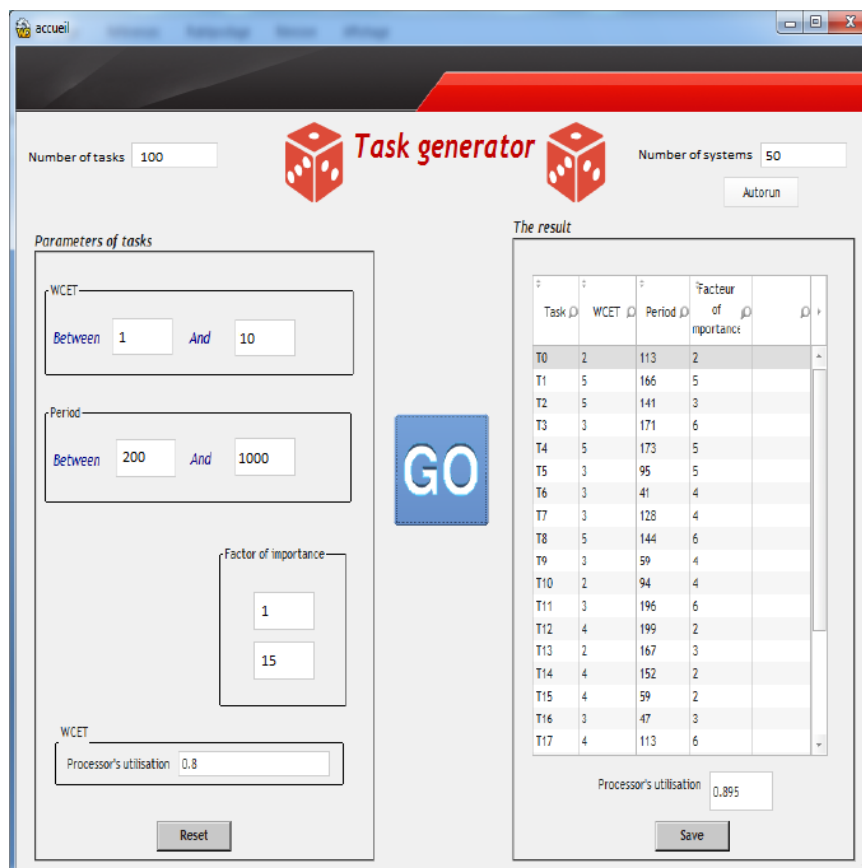
FIGURE 3.16: Interface graphique du module de génération aléatoire Task-generator .
