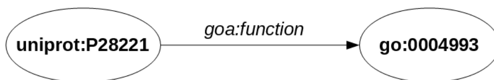
FIGURE 1.6 – Représentation en graphe du triplet uniprot:P28221 goa:fonction go:0004993 , représentant l'annotation de la protéine P28211 par la fonction GO serotonin receptor activity ( go:0004993 ). Ici les URIs utilisent une notation préfixée, telle que uniprot:P28221 correspond à l'URI http://bio2rdf.org/uniprot:P28221 , goa:fonction correspond à http://bio2rdf.org/goa_vocabulary:fonction et go:0004993 correspond à http://bio2rdf.org/go:0004993 .
