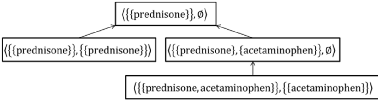
FIGURE 2.1 – Représentation des données de la Table 2.2 dans un semi-treillis construit à partir de la structure de patrons (G, (\mathcal{D}_1, \sqcap_1), \delta_1) , où les flèches représentent l'ordre partiel \leq_{\sqcap_1} défini par \sqcap_1 .
