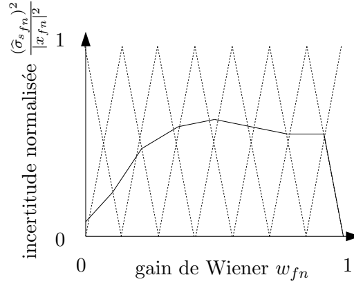
Figure 1.4: E = 8 fonctions noyaux triangulaires b^e(w_{fn}) (traits pointillés) et estimateur non-paramétrique de l'incertitude (\hat{\sigma}_{s_{fn}}^{\text{fus}})^2/|x_{fn}|^2 (trait plein). L'axe horizontal représente la proportion de parole dans le spectre de puissance de la parole bruitée observé. L'axe vertical est proportionnel à l'incertitude. L'incertitude est normalisée par le spectre de puissance de la parole bruitée pour illustrer le fait que la forme de l'estimateur (le trait plein) n'en dépend pas. Le trait plein est obtenu en sommant les traits pointillés avec différents poids positifs.
