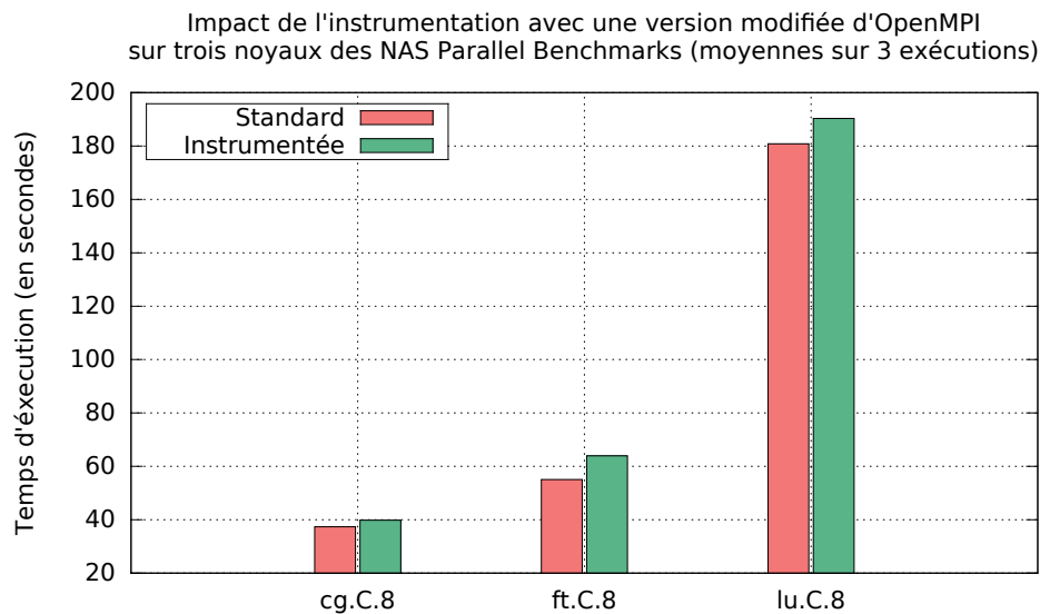
Figure 2.3 – Évaluation de l'impact de l'instrumentation des communications avec une version modifiée de Open MPI sur des noyaux des NAS en classe C sur 8 processeurs. Les expériences ont été réalisées sur un nœud PlaFRIM embarquant un processeur Intel Xeon X5550.
