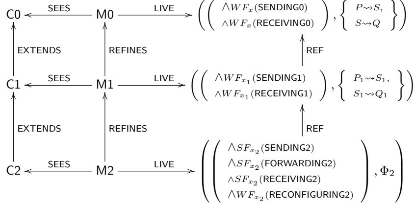
FIGURE 6.22 – Deuxième raffinement du NoC
