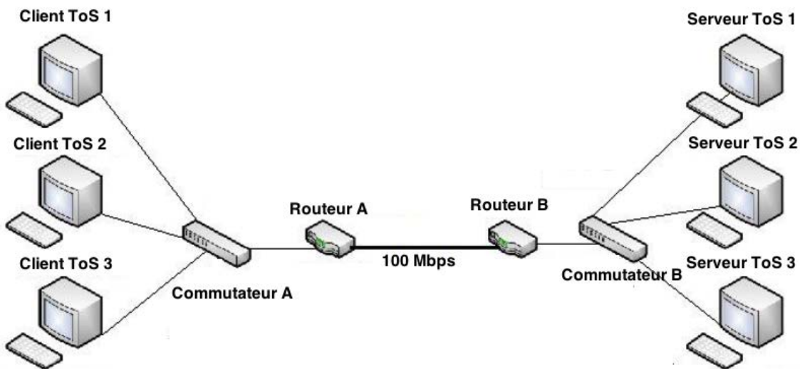
FIGURE 5.6 – Scénario de capture de la trace simulée avec OPNET
