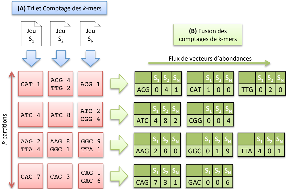
FIGURE 3.3. Stratégie de comptage de k -mers multi-jeu avec k=3 . (A) Un processus de comptage, représenté par une flèche bleue, compte les k -mers d'un jeu de données indépendamment des autres. Chaque processus produit une colonne de P partitions (carrés rouges) contenant des k -mers triés et leurs comptages. (B) Un processus de fusion, représenté par une flèche verte, fusionne une ligne de N partitions. Il produit des vecteurs d'abondances, représentés en vert, qui nourrissent l'étape de calcul des distances.
