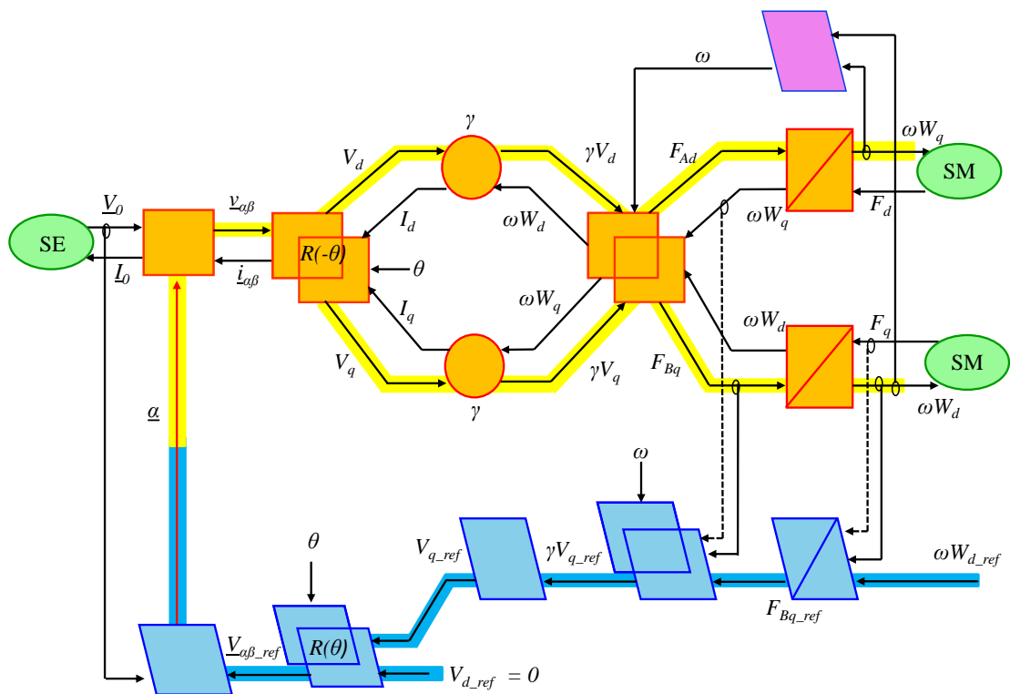
FIGURE C.5: REM de l'asservissement de l'amplitude vibratoire et de la fréquence de résonance du transducteur de Langevin dans un repère tournant
