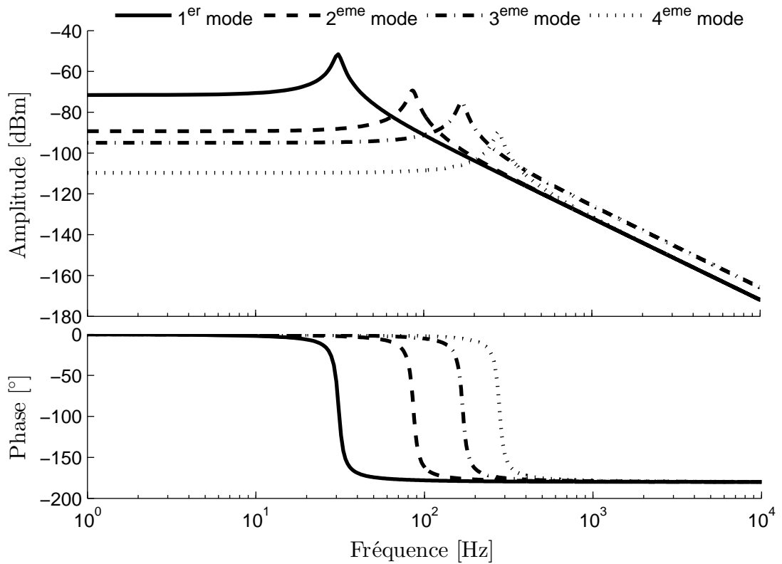
FIGURE 2.10: Amplitudes et phases des quatre premiers modes de vibration d'une poutre en aluminium 350 \times 6 \times 6 \text{ mm}^3 excitée par une force de 1 N
