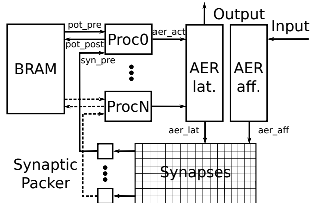
FIGURE 2.11 – Architecture utilisant les blocs mémoire du FPGA afin de multiplexer le calcul neuronal. Les événements d’entrées et latéraux sont intégrés dans la grille de synapses. Plusieurs processeurs parallèles effectuent la mise à jour du potentiel de chaque neurone avec une précision de 18 bits en lisant et en écrivant dans un bloc mémoire et en lisant les potentiels synaptiques.
