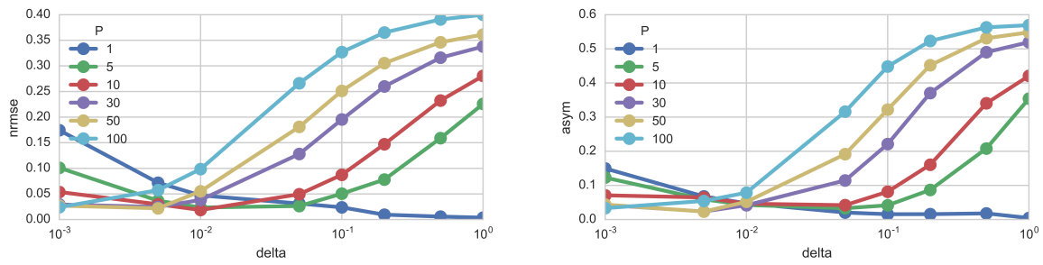
FIGURE 4.6 – Biais de propagation des flux de bits. Haut : la NRMSE en fonction de \delta et du nombre d’activations P . Bas : l’asymétrie entre le nombre de bits reçus par les neurones situés dans la colonne du milieu et ceux situés dans la ligne du milieu. N = 10000 .
