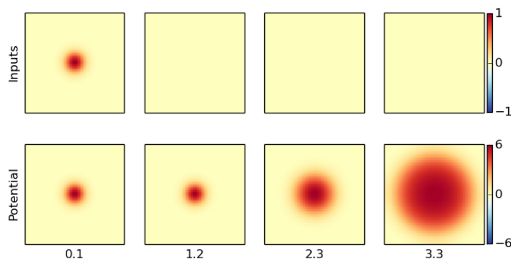
FIGURE 1.7 – Fronts progressifs (bas) après une impulsion de 1.2s (haut).
