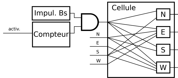
FIGURE 4.10 – Diagramme de la cellule CASAS et du flux de bits impulsionnel associé. Lorsque le neurone est activé, un compteur active le flux de bits impulsionnel pour la longueur des flux de bits désirée. Les impulsions entrantes sont routées avec les quatre routeurs nord (N), est (E), sud (S) et ouest (W).
