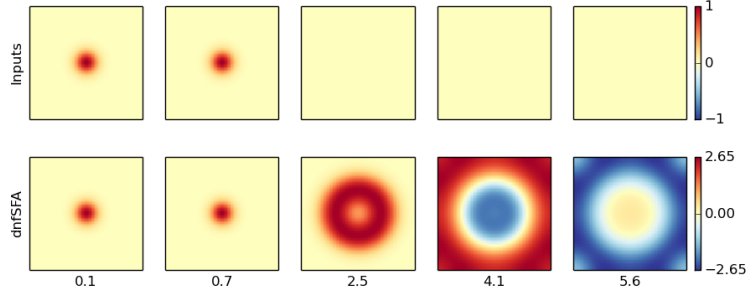
FIGURE 1.8 – Vague progressive. Une impulsion de 1s (haut) provoque une vague d’excitation suivie d’une vague d’inhibition dans les potentiels membranaires des neurones (bas).
