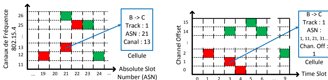
(a) Le multiplexage FTDM sur IEEE Std 802.15.4-2015 mode TSCH à 2.4 GHz (b) Un échancier pour IEEE Std 802.15.4-2015 mode TSCH à 2.4 GHz
