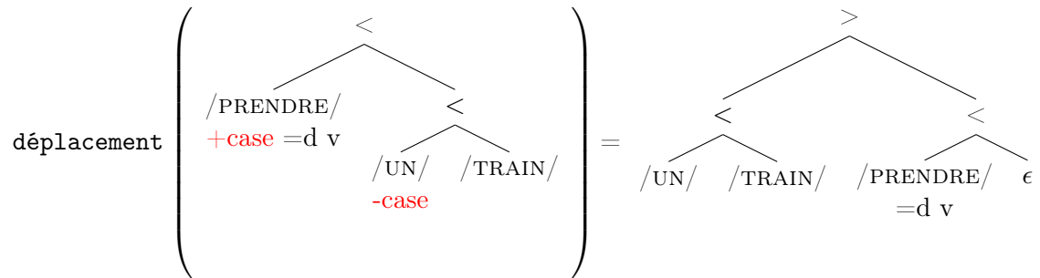
FIGURE 2.2 – Exemple d’application des règles de fusion et de déplacement dans les MG de Stabler
