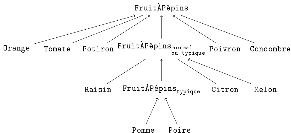
FIGURE 6.3 – Réorganisation de la hiérarchie des aliments dont la racine est FruitÀPépkins par la méthode des seuils.
