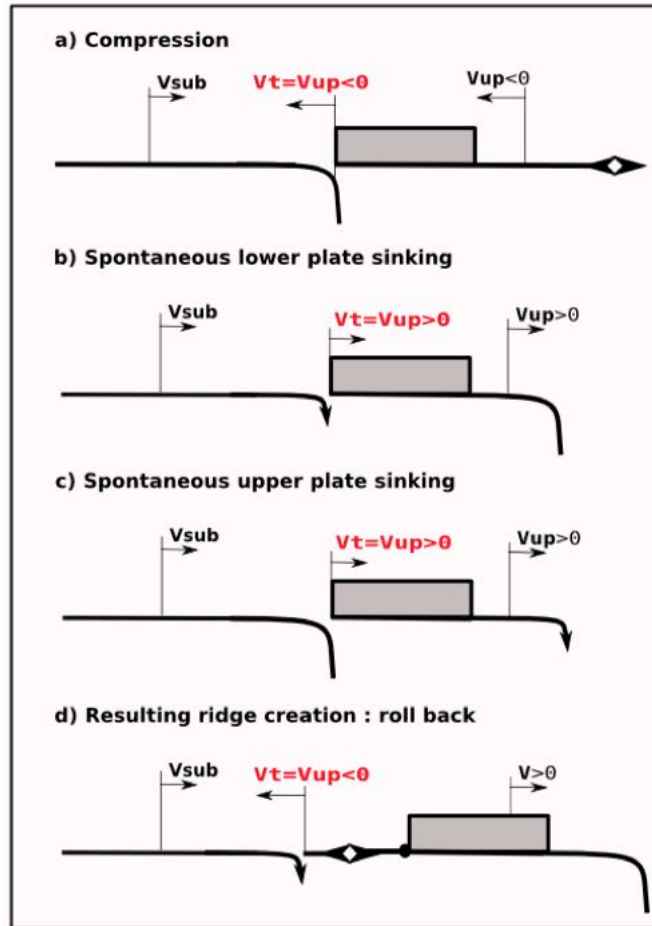
FIGURE 2.6 – Comportement des fosses de subduction basé sur un critère structurel – Les vitesses sont comptées positivement dans le sens de déplacement de la plaque plongeante. a) Si la plaque supérieure ne possède pas de slab , le régime est considéré comme compressif, et la migration de la fosse est prescrite par le mouvement de la plaque supérieure : V_t = V_{up} . Si au contraire la plaque supérieure est entraînée par un slab pull , elle s'éloigne rapidement de la fosse et le régime est considéré comme extensif. Ceci a lieu en cas d'initiation d'une subduction (b) pour la plaque inférieure ou (c) pour la plaque supérieure. Dans les deux cas, une dorsale océanique est créée devant la fosse qui sépare les deux plaques, et le plancher nouvellement formé est suturé sur l'ancienne plaque supérieure, tandis que de l'autre côté, la plaque plongeante part en roll-back suivant V_t = V_{up} (d)
