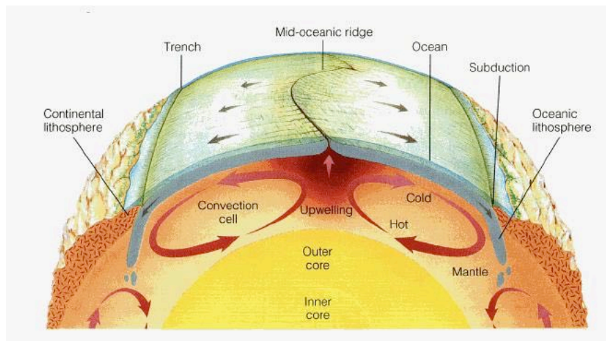
FIGURE 2.2 – Schéma simplifié du couplage entre plaques tectoniques et manteau convectif – Les cellules de convection du manteau sont bornées par des courants chauds ascendants à l'aplomb des dorsales, et des courants froids descendants au niveau des zones de subduction. Source : http://www.planet-terre.ens-lyon.fr
