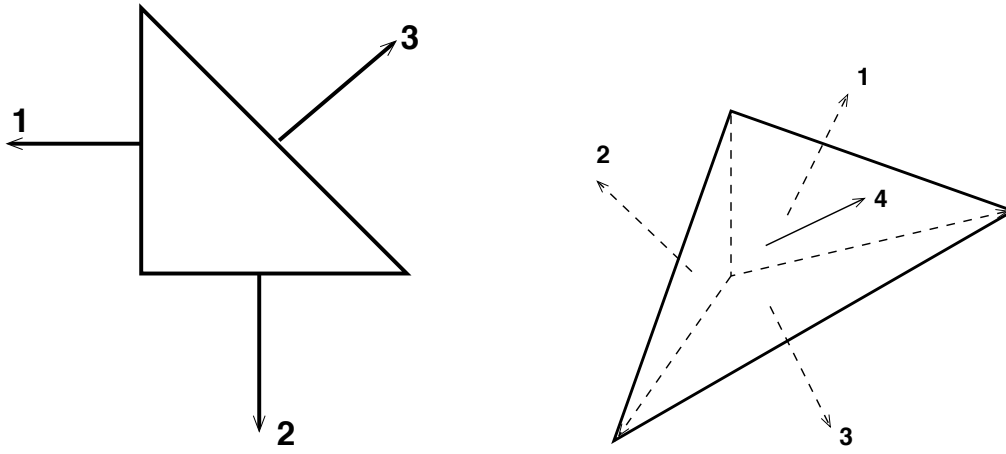
FIGURE 3.1 – Elément fini de Raviart-Thomas \mathbb{RT}^0 en dimension 2 (gauche) et 3 (droite).
