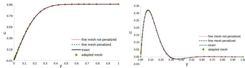
FIGURE 6.29 – Profil de la composante U de la vitesse pour les différents maillages. A gauche : vitesse constante ; à droite : vitesse oscillante.
