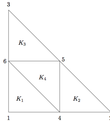
FIGURE 6.34 – Triangle subdivisé pour la p-adaptation
