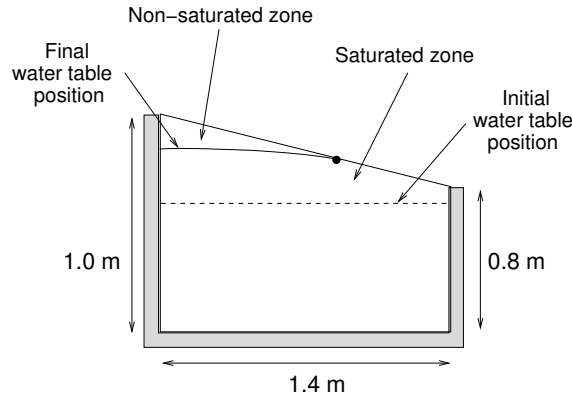
FIGURE 1.2 – Géoétrie d'Abdul et Gillham.
