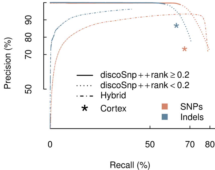
FIGURE 2.13 – Résultats de détection d’indels et de SNP sur des données simulées provenant du chromosome 1 humain. Les courbes de précision par rapport au recall sont obtenues en classant les prédictions par rapport à leur score \Phi pour discoSnp++ (voir Section 2.7.4 page 31) ou par rapport à leur score fourni par GATK pour l’approche hybride. Les lignes pointillées des résultats discoSnp++ concernent les prédictions pour lesquelles \Phi < 0.2 .
