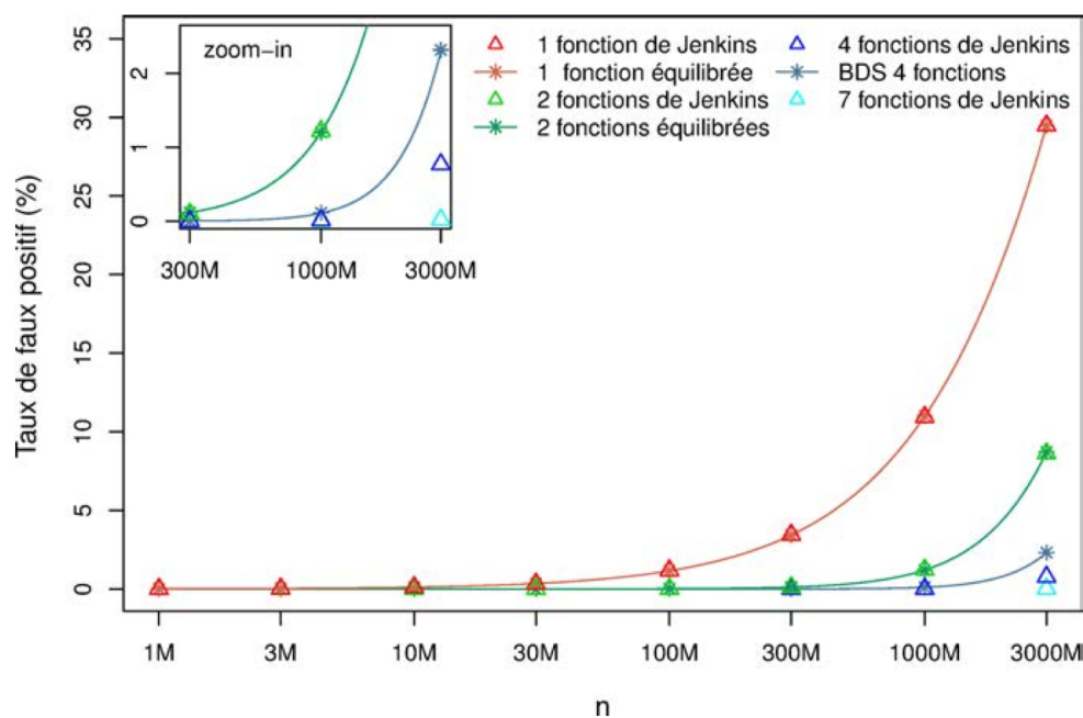
FIGURE 3.3 – Image tirée de [Maillet, 2013]. Taux de faux positifs en fonction de la méthode d'indexation utilisée et du nombre de mots indexés ( n ). La courbe “BDS 4 fonctions” est la solution utilisée dans les méthodes développées.
