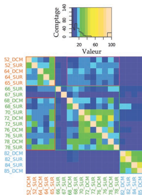
FIGURE 3.10 – Heat map des intersections de 13 stations de Tara Oceans pour des organismes d'une taille de 180 \mu\text{m} à 2000 \mu\text{m} . Le code couleur est donné dans la légende de la Figure 3.9 page ci-contre. De plus, le rectangle délimité en rouge représente le pourcentage de séquences de l'océan atlantique sud similaires à des séquences de l'océan indien. Le rectangle délimité en mauve représente le pourcentage de séquences de l'océan indien similaires à des séquences de l'océan atlantique sud.
