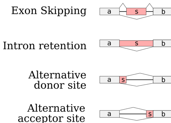
FIGURE 2.5 – Impage importée de [Sacomoto et al., 2012]. Représentation de différents scénarios d’épissage alternatif. L’“exon skipping” indique qu’un exon peut être entièrement épissé. L’“intron retention” indique qu’un intron est entièrement conservé dans l’ARNm. Les cas “alternative donor site” et “alternative acceptor site” indiquent une coupure exon/intron (respectivement une coupure intron/exon) alternative.
