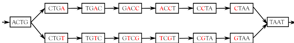
FIGURE 2.9 – Représentation d'une bulle générée par la présence de SNPs proches dans un DBG. Dans cet exemple, k = 4 et les données contiennent les séquences ACTGACCTAAT et ACTGTCGTAAT.
