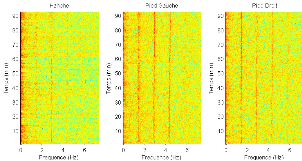
Figure 3.12 – Spectrogramme de chaque lien durant la course, montrant l'évolution temporelle de la densité spectrale de puissance. La périodicité des effets du masquage lié au mouvement régulier de course est mise en évidence par la combinaison principale de trois fréquences, correspondant à la fréquence de foulée (fondamentale) et ses deux premières harmoniques.
