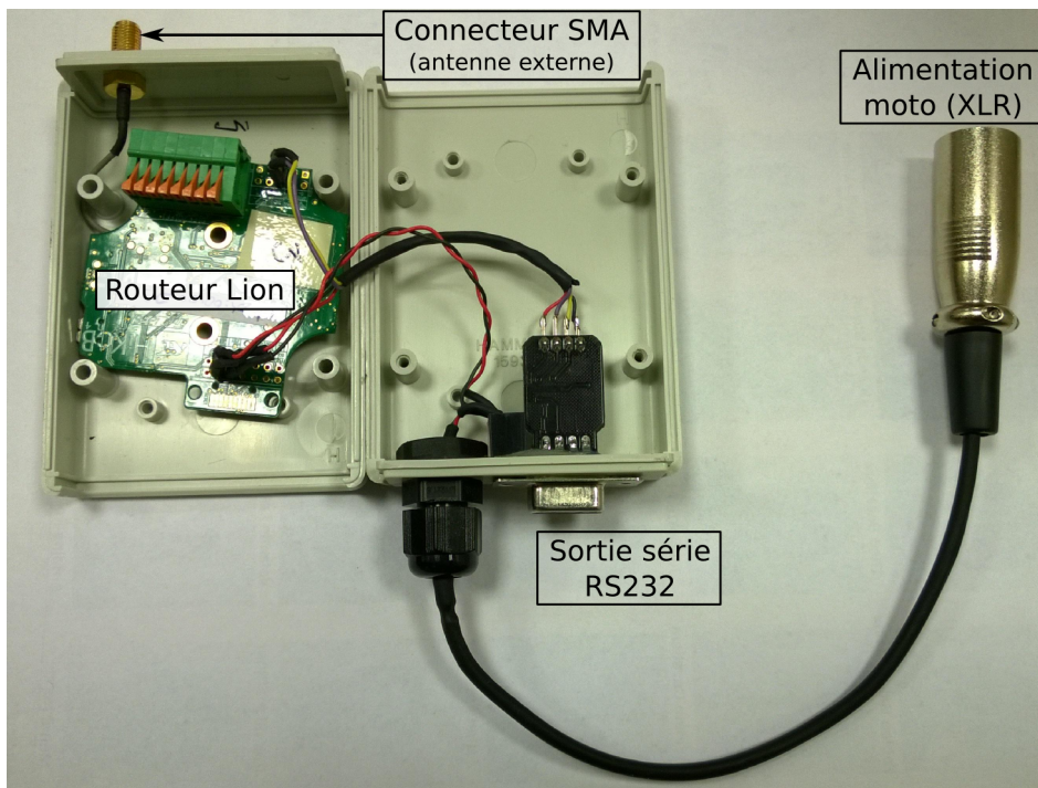
Figure 2.6 – Photo d'un routeur Lion dans son boîtier, tel qu'embarqué dans les motos, avec la connectique permettant de s'interfacer avec le système Euromedia.
