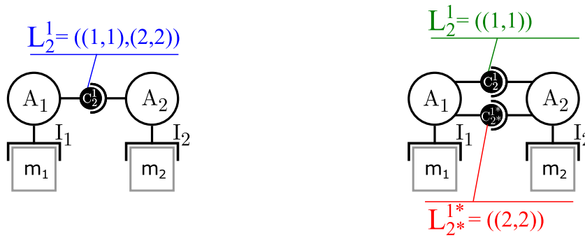
(a) Exemple de multi-modèle AA4MM.
