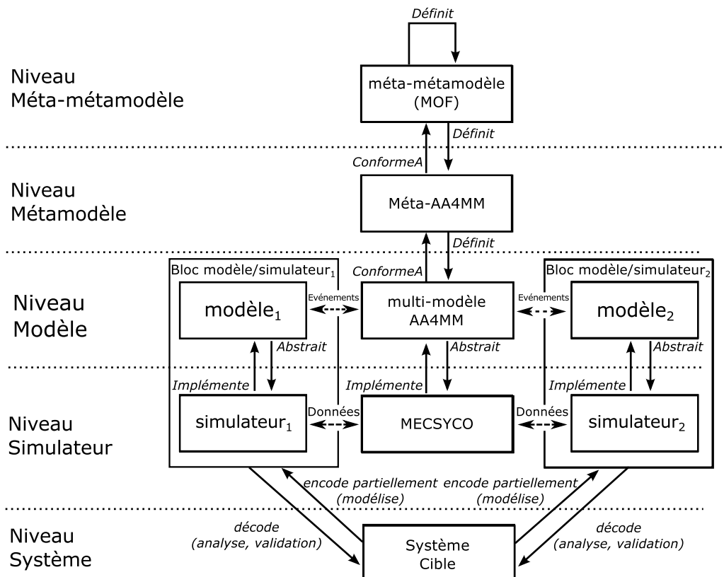
FIGURE 7.3 – L'approche d'ingénierie dirigée par les modèles pour AA4MM ( les relations entre le système cible et les blocs modèle/simulateur sont inspirées de [Seck and Honig, 2012]).
