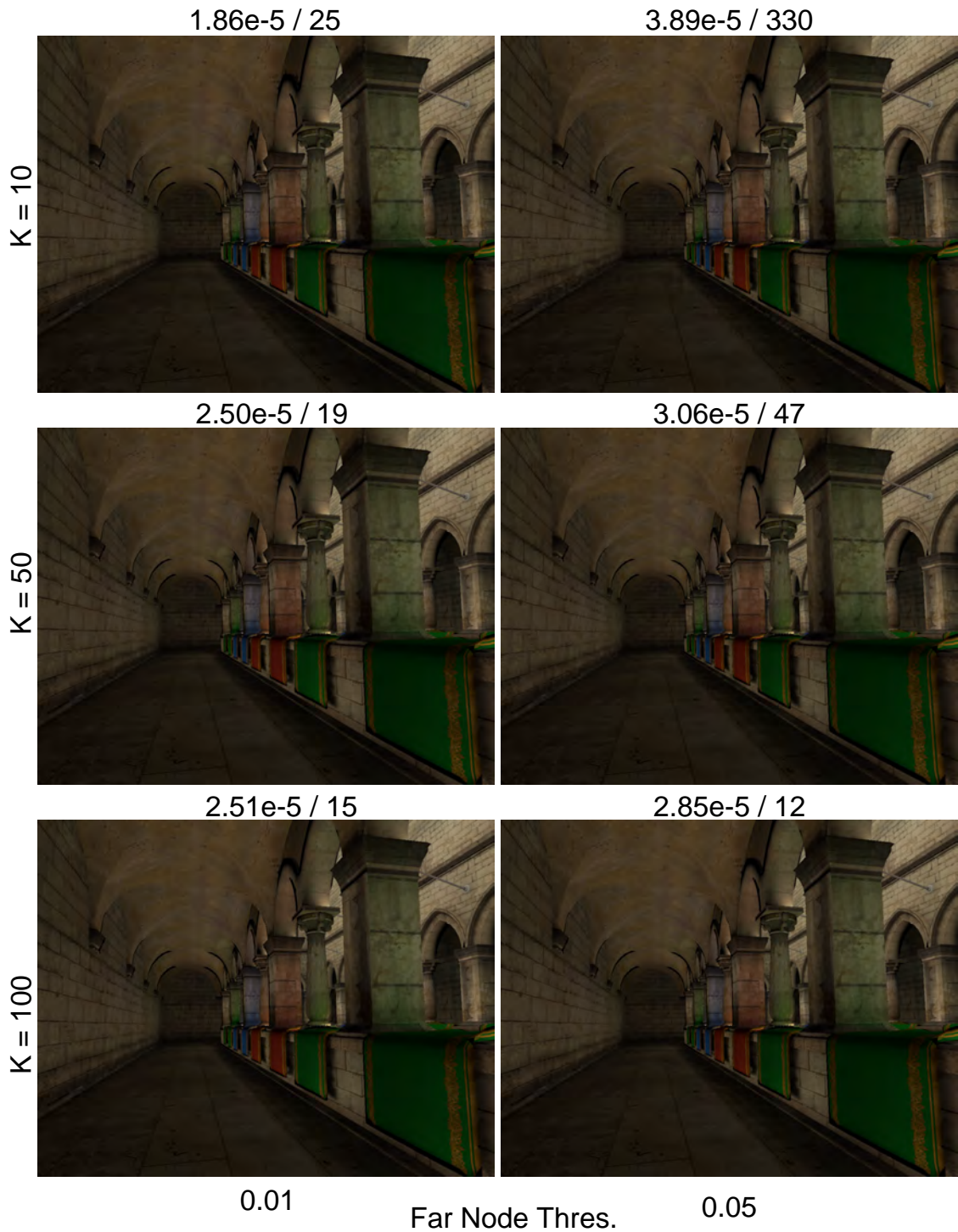
图 3.13 参数分析: 在不同参数下的渲染结果, 以及与 PBGI 算法进行对比的误差值<MSE>/<PDP>。
