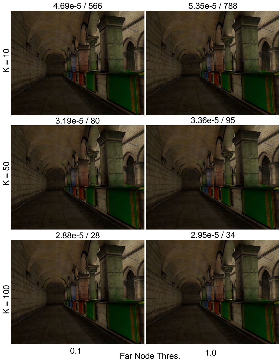
图 3.14 参数分析(续): 在不同参数下的渲染结果, 以及与 PBGI 算法进行对比的误差值<MSE>/<PDP>。
