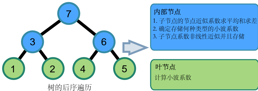
图 4.7 为了避免整个点云的小波系数都存在内存中，我们采用后序遍历的方式，on-the-fly 模式计算点云的小波系数：计算子节点的小波系数并且进行和平均、差平均，对于子节点决定存储何种小波系数，进行非线性近似并且存储。
