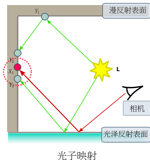
图 1.8 光子映射算法。该算法分为两部分：第一部分，由光源发射光子，与场景相交和反弹，存储与非镜面反射表面的交点形成光子图，如绿色圆圈所示；第二部分，从相机发射光线，计算出第一个非镜面的交点(该过程表示为红色)，通过对光子图查找(比如最近邻算法)计算出该交点的辐射亮度。
