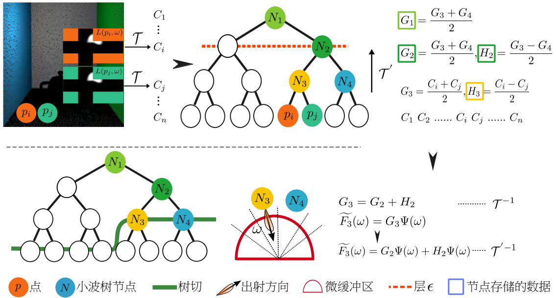
图 4.4 算法流程。首先，对场景采样得到点云，将点云组织到点云层次结构，并且采用后序遍历来计算每个节点/点的小波系数。对于叶节点/点，将其直接光照按照立方体贴图采样，然后对立方体贴图的每个面进行哈尔小波变换 ( \mathcal{T} ) 从而得到系数向量 C_i ；计算中间节点的辐射亮度分布，对子节点小波系数进行小波分析 ( \mathcal{T}' ，或者说求和平均和求差平均)，从而得到两种系数类型，节点近似系数 G 和细节系数 H 。树中小于(靠近根节点)层 \epsilon (红色虚线)的节点只存储近似系数，层数大于(靠近叶节点) \epsilon 的节点只存储细节系数，该层上的节点存储两者；计算着色点的间接光照时，遍历点云树，将节点投影到微缓冲区中，首先计算出节点近似系数(大于 \epsilon 层的节点)，然后，重构出节点的辐射亮度。
