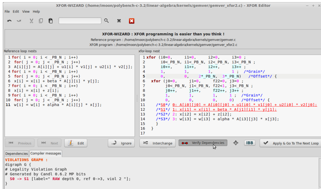
Figure 6 – XFOR-WIZARD : L'Éditeur XFOR.
