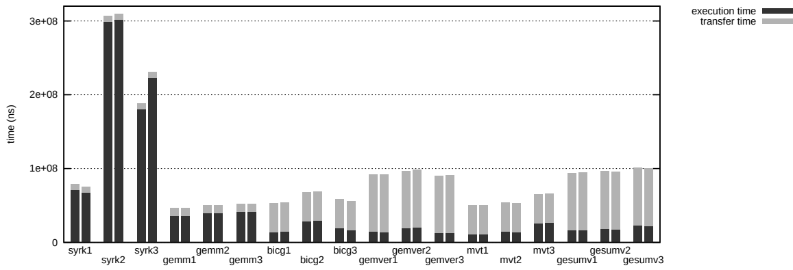
FIGURE 1.2 – Comparaison entre temps d’exécution prédit (barre gauche) et effectif (barre droite) sur PolyBench avec le jeu de données standard sur GTX 590.
