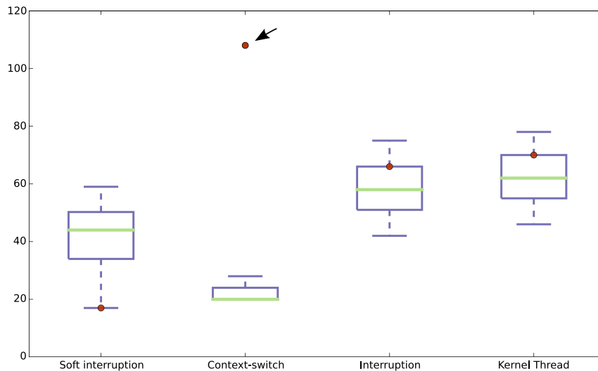
FIGURE 5.24 – Description des régimes irréguliers à l’aide des boîtes à moustaches : les boîtes à moustaches représentent la distribution des certains événements dans un régime régulier et les points représentent le nombre d’occurrences de ces événements dans le cas d’un régime irrégulier détecté.
