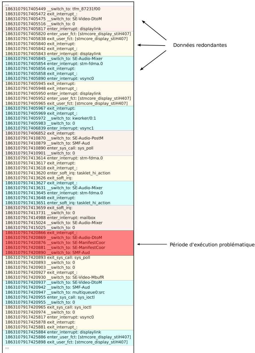
FIGURE 1.2 – Illustration des régimes de fonctionnement répétitifs et problématiques présents dans la trace d'exécution d'une application.
