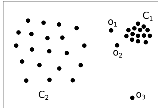
FIGURE 3.2 – Les anomalies globales et locales : o_1 et o_2 sont des anomalies locales, o_3 est une anomalie globale
