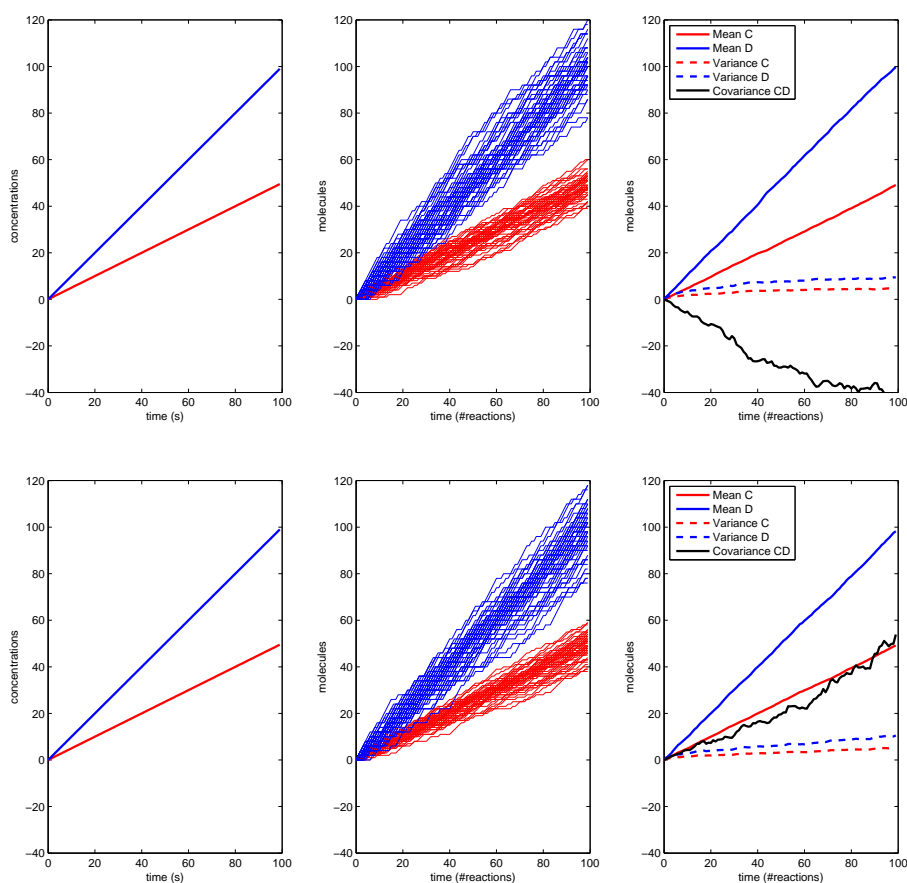
FIG. 1 – Réseaux distinguables par leurs moments d'ordre 2 Dynamiques différentielles et stochastiques pour le modèle 1 (première ligne) et le modèle 2 (seconde ligne) décrits dans Eq. (3). Les courbes rouges (resp. bleues) représentent les quantités de C (resp. D). La première colonne représente la solution de l'équation différentielle issue de la loi d'action de masses. La seconde colonne représente 50 générations de trajectoires aléatoires obtenues à l'aide d'un algorithme de simulation stochastique. Les paramètres cinétiques et stochastiques ont été fixés à 1 et il y a 1000A et 1000B initialement. La troisième colonne représente les estimations des espérances, des variances et des covariances croisées entre C et D . Ces estimations sont obtenues à partir des 50 trajectoires de la seconde colonne. On constate que seule la trajectoire des covariances de C et D permettent de distinguer ces réseaux.
