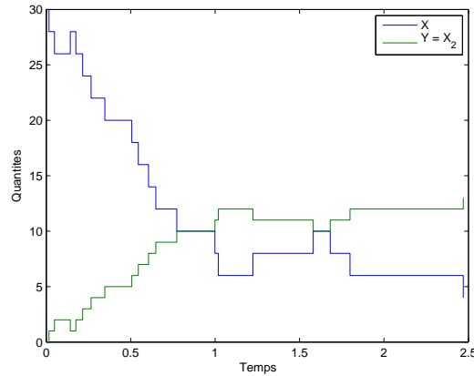
FIG. 3.2 – Simulation de Gillespie du réseau de dimérisation pour a_0 = 15 , c_1 = c_2 = 0, 1 .
