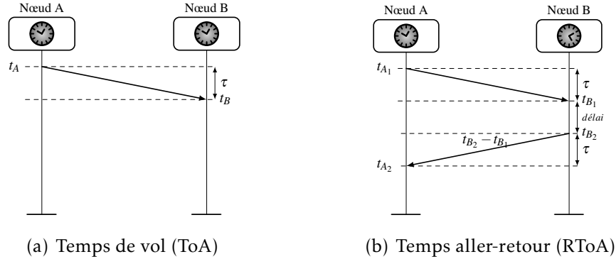
FIGURE 1.5 – Télémétrie avec des mesures de temps.
