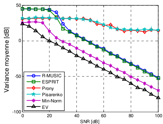
Figure VI.4 Variance moyenne de l'estimation fréquentielle des barres rotoriques cassées
