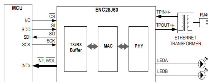
Figure III.3 Interconnexion entre le circuit d'Ethernet et le MCU
