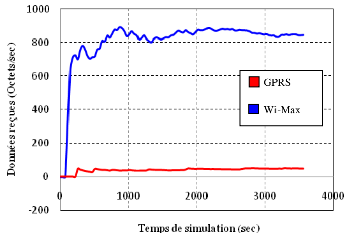
Figure III.16 Trafic moyen reçu avec le service HTTP
