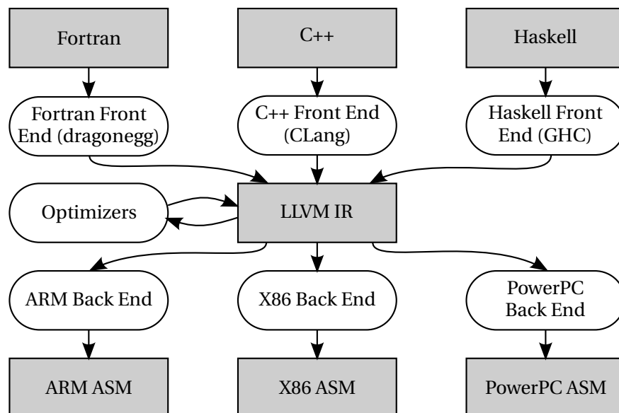
FIGURE 4.8 – Vue d'ensemble du flux de compilation LLVM.
