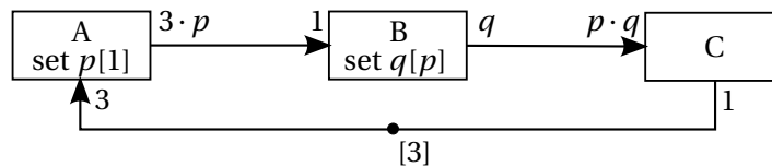
FIGURE 3.5 – Exemple de graphe SPDF
