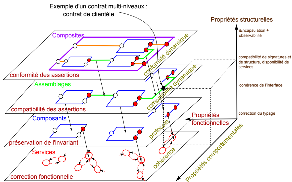
FIGURE 5.1 – Différents aspects de la modélisation des systèmes à base de composants.
