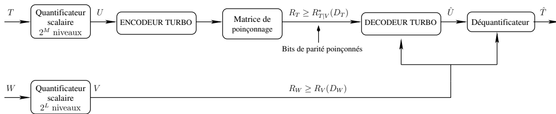
FIG. 3.15 – Système de codage distribué de deux sources quantifiées utilisant un code turbo poinçonné.
