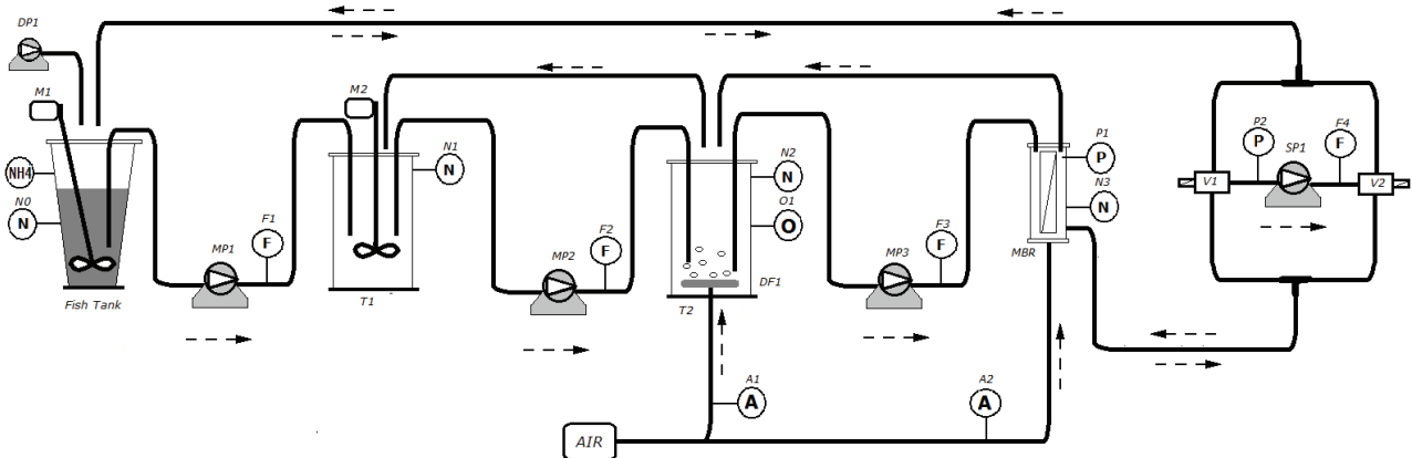
Figure 3: Schéma des systèmes d'aquaculture de recirculation équipé d'un BRMS.
