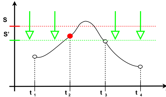
Figure 0.1: Le processus discrétisé rate le seuil mais S mais pas le seuil S' .
