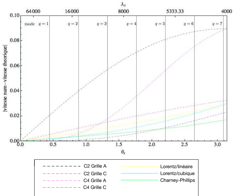
FIGURE 2.7 – Erreur de déphasage |c_{\text{num}} - c_{\text{th}}| en fonction de \theta_x \in [0; \pi] . La discrétisation horizontale étant fixée ( \Delta x = 2000\text{m} ), on retrouve la longueur d'onde correspondante ( \lambda_x en m ). Les longueurs d'onde correspondant aux différents modes q sont indiqués.
