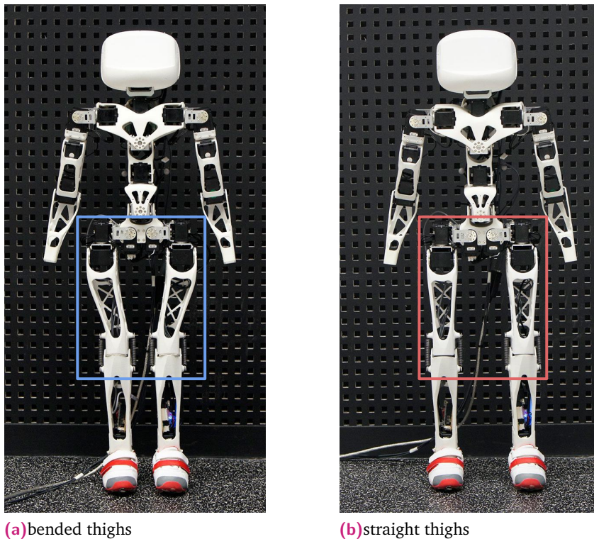
Fig. 0.2.: Exemple de modification de la morphologie de Poppy. Ici l'architecture modulaire permet de remplacer les cuisses de Poppy et de comparer 2 configurations, une bio-inspirée (à gauche) et une plus traditionnelle (à droite)
