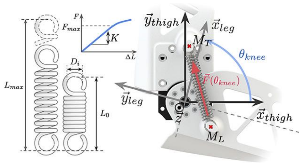
Fig. B.1.: Spring parameters to optimize
